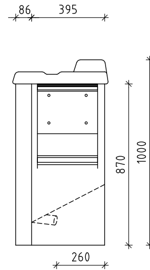
Seitenansicht Mattenablage
