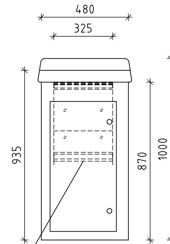
Seitenansicht Türseite
