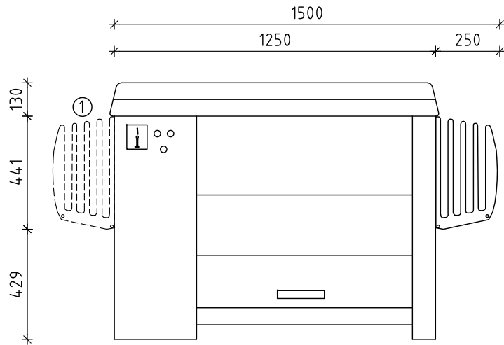
Ansicht Frontseite
